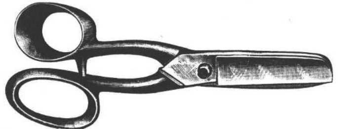
Art. 610 Lederschere mit Zahnung , extra starke gerade Ausführung, mit kräftigen Schenkeln Normallänge ca. 220 mm .....
